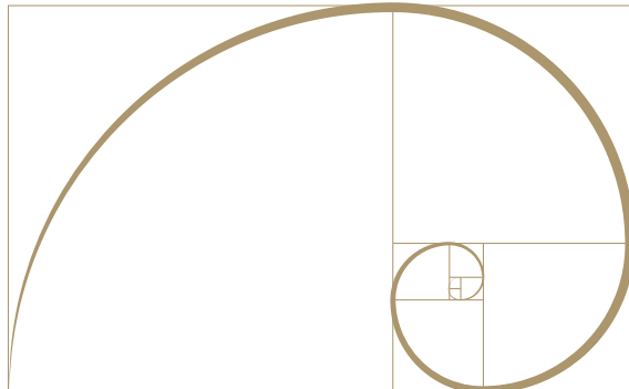
Le nombre d'or
