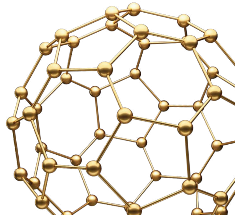
La molécule Fullerène C_{60}
